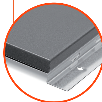
Luftschlitze zur aktiven Hinterlüftung Die seitlich eingebrachten Luftschlitze sorgen in Kombination mit dem rückseitigen Abstand der Heizung zur Tischplatte für einen permanenten Luftaustausch. So wird die Tischplatte niemals zu heiß.
